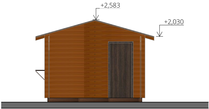
Severní pohled (M 1:75)
