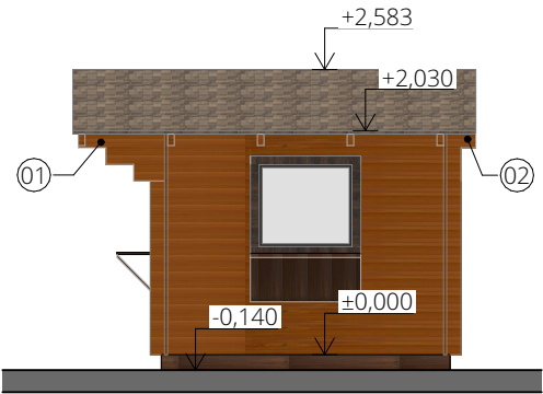
Východní pohled (M 1:75)
