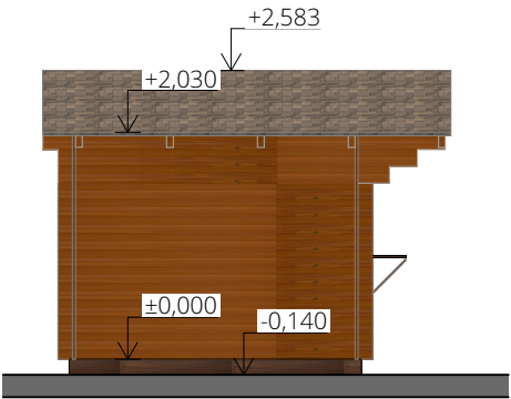
Západní pohled (M 1:75)
