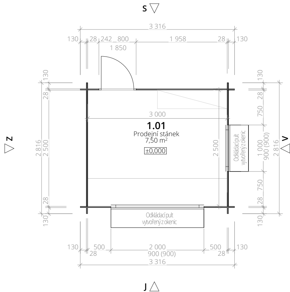
Půdorys (M 1:50)
